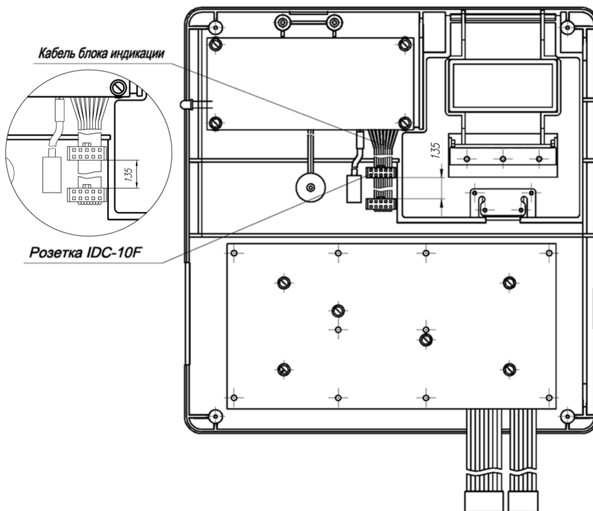
Рисунок 5 – Модернизация верхнего корпуса
